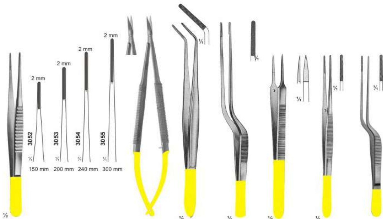
3051 DE BAKAY 17,5 cm
